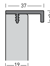
Sezione anta Door section
