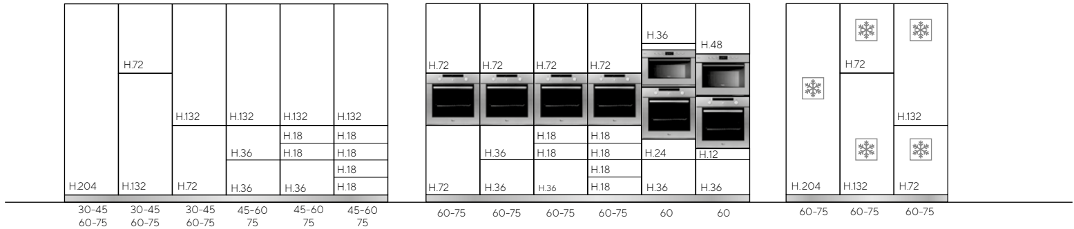
Colonne frigorifero H. 132 Tall units for refrigerator H. 132
