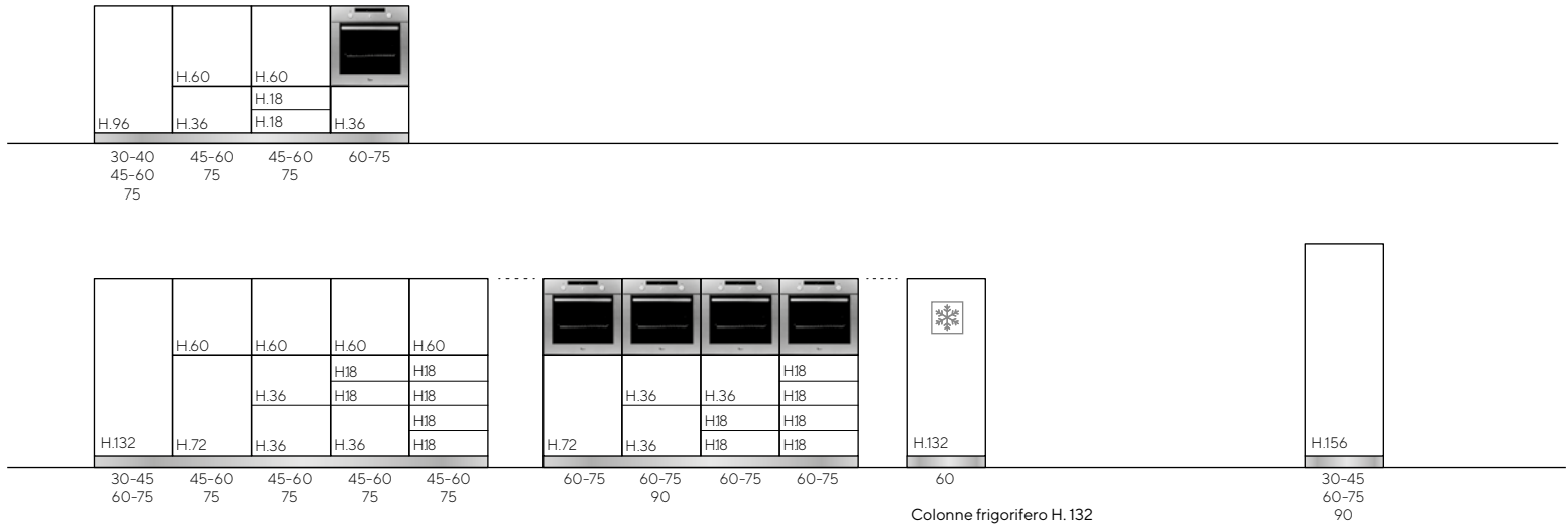
Colonne frigorifero H. 132 Tall units for refrigerator H. 132
