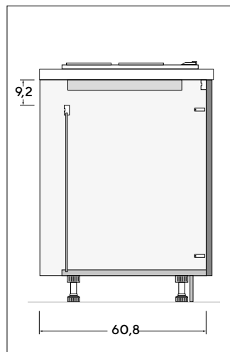
Sezione base piano cottura H.72 con apertura maniglia H..72 hob base unit section with handle opening
