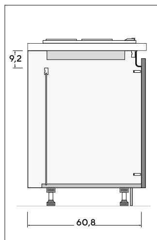
Sezione base piano cottura H.75 con apertura gola H.75 hob base unit section with groove opening
