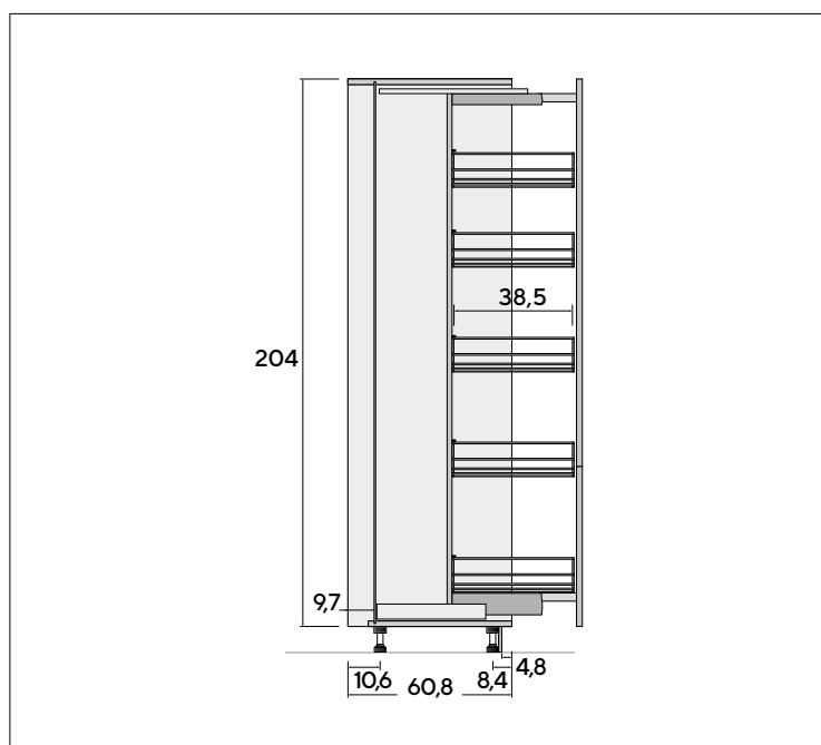
Cesti estraibili Extractible baskets
