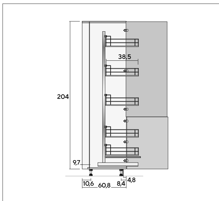
Cesti estraibili Maxi Maxi extractible baskets
