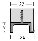
Sezione ante Door section
